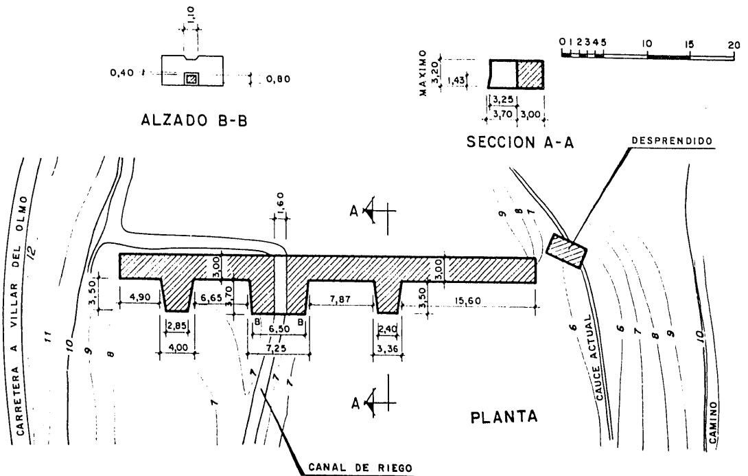
Presa sobre el arroyo Vega, en Ambite (Madrid).
