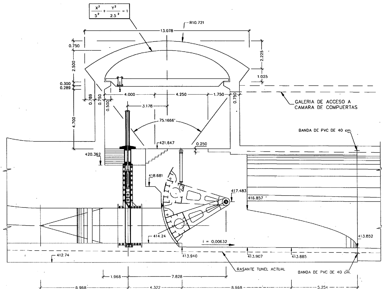
Figura 7. Cámara de compuertas. Sección longitudinal.
