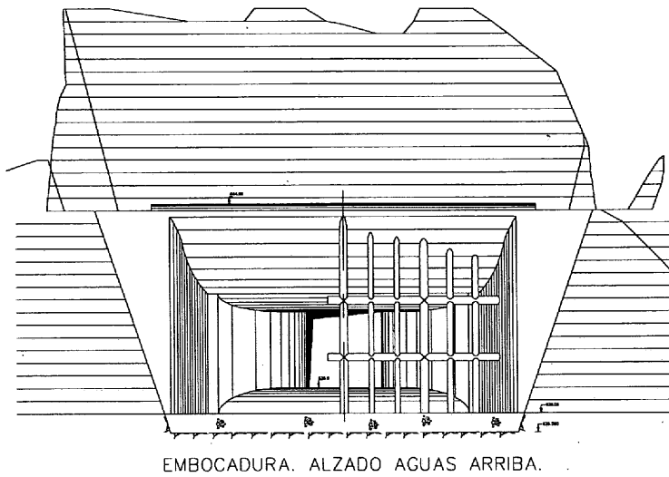
Figura 2. Embocadura. Alzado y secciones.
