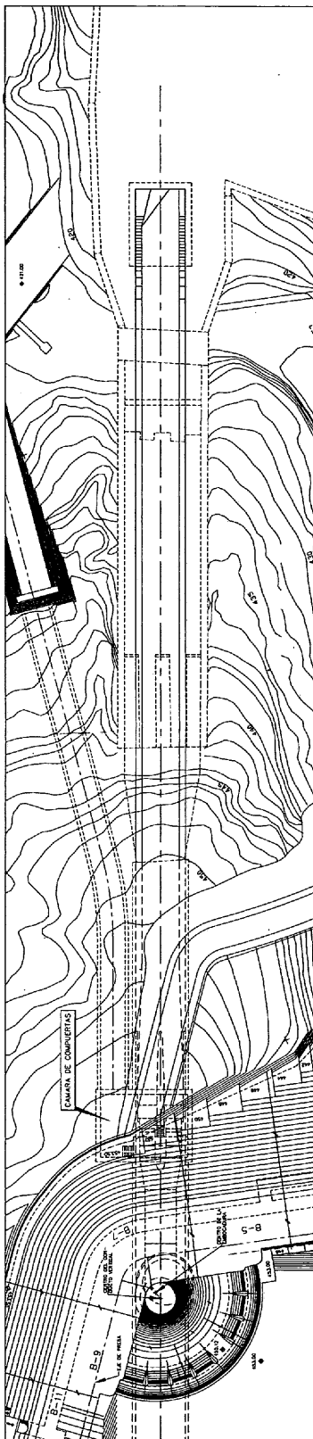
DESAGÜE DE MEDIO FONDO PLANTA GENERAL
