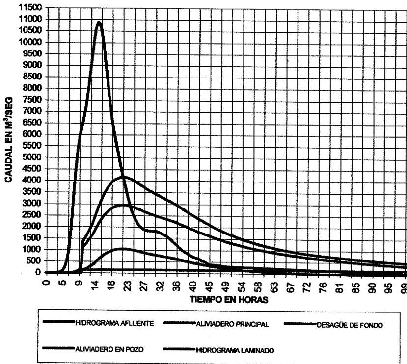
PRESA DE CONTRERAS CON MORNING GLORY LAMINACIÓN DE LA AVENIDA MÁXIMA PROBABLE
