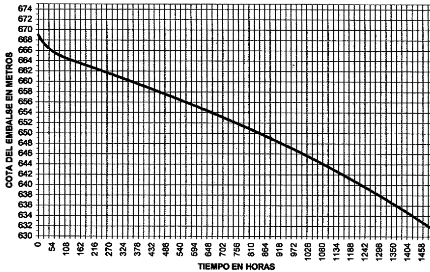
Gráfico 5. Contreras. Vaciado del embalse. "Morning Glory".
