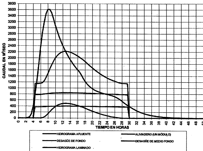
NUEVA PRESA DE PUENTES LAMINACIÓN DE LA AVENIDA DE 1000 AÑOS
