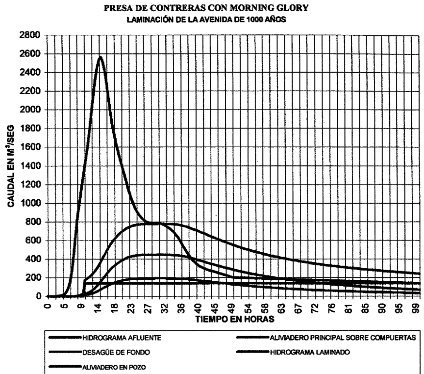
Gráfico 1. Contreras. Avenida de 1.000 años. "Morning Glory".
