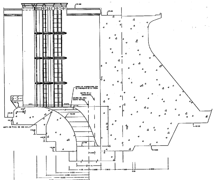
Figura 6. Embocadura. Sección.
