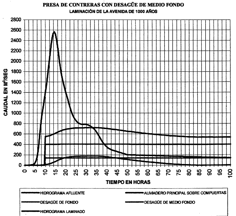
Gráfico 2. Contreras. Avenida de 1.000 años. Desagüe de Medio Fondo.
