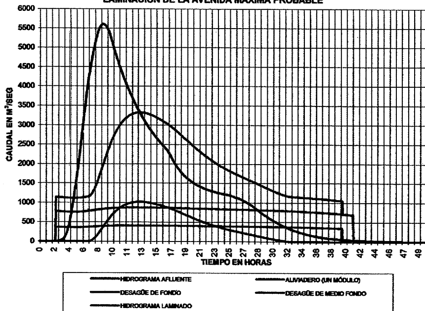
NUEVA PRESA DE PUENTES LAMINACIÓN DE LA AVENIDA MÁXIMA PROBABLE
