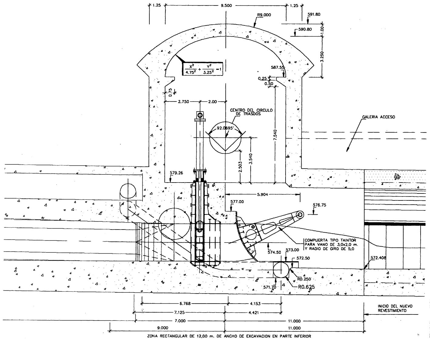
Figura 3. Cámara de compuertas. sección longitudinal.
