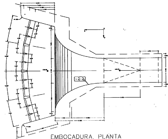
EMBOCADURA. PLANTA DEFINICION GEOMETRICA.
