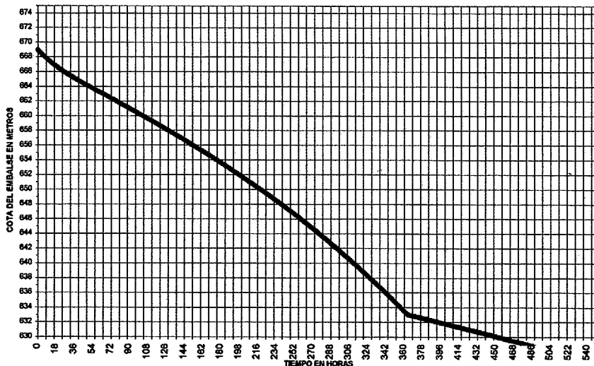
PRESA DE CONTRERAS CON DESAGÜE DE MEDIO FONDO VACIADO DEL EMBALSE
