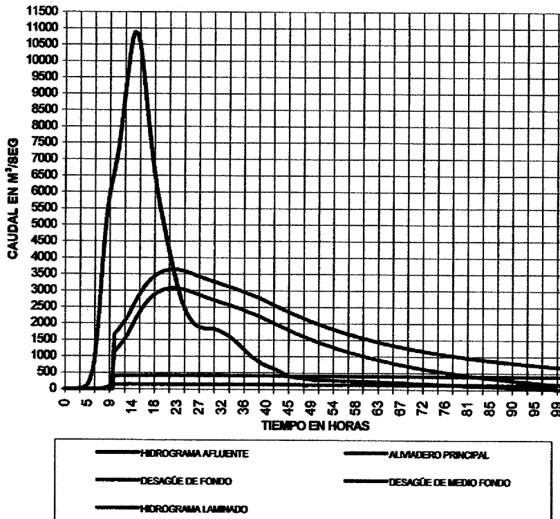
PRESA DE CONTRERAS CON DESAGÜE DE MEDIO FONDO LAMINACIÓN DE LA AVENIDA MÁXIMA PROBABLE
