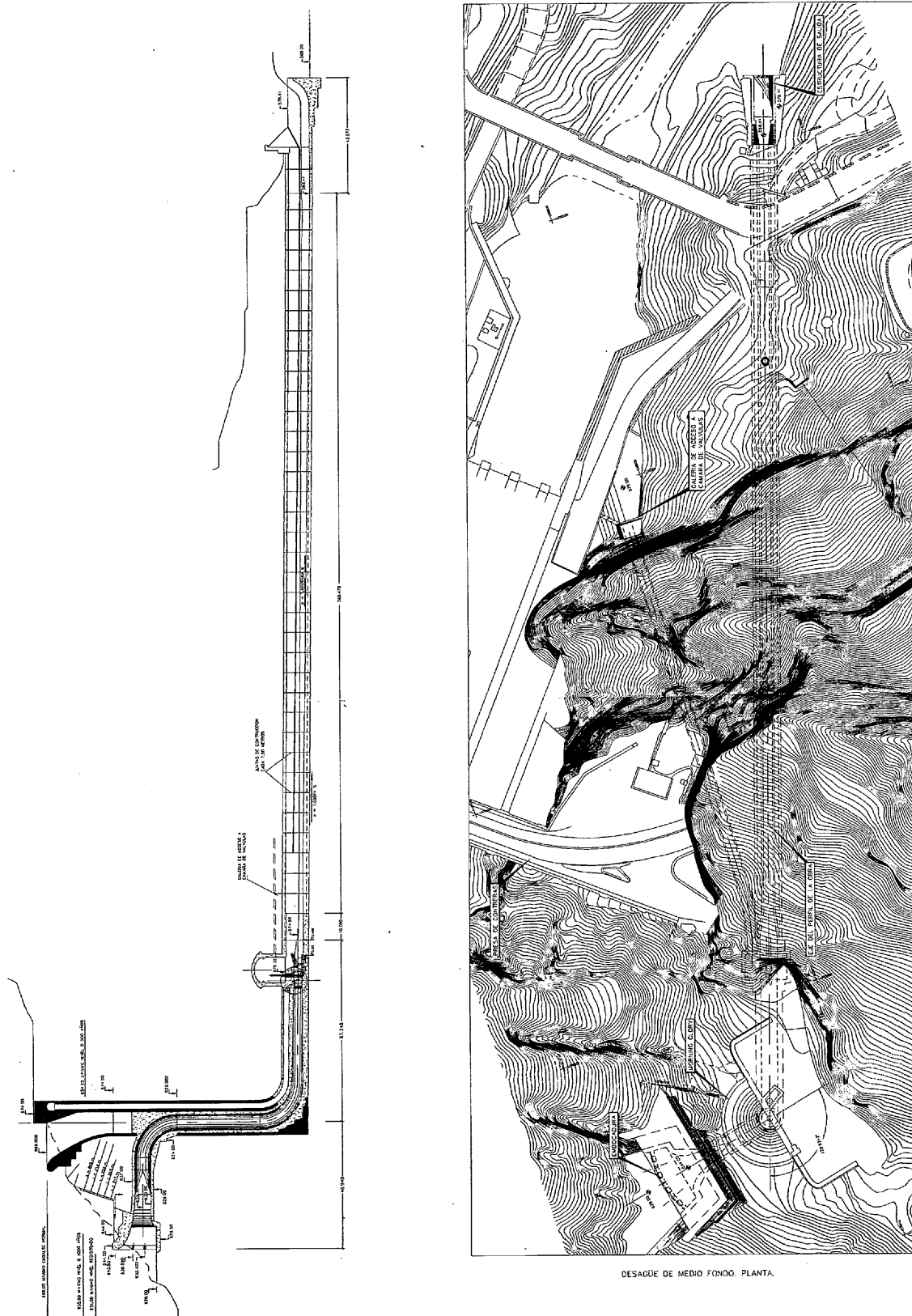
DESAGÜE DE MEDIO FONDO. SECCION LONGITUDINAL POR EL EJE.
