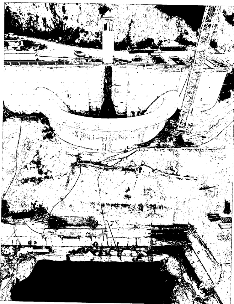
Foto 1. Presa de Contreras. Vista del Caliz del actual "morning glory" y excavación del futuro desagüe de medio fondo.
