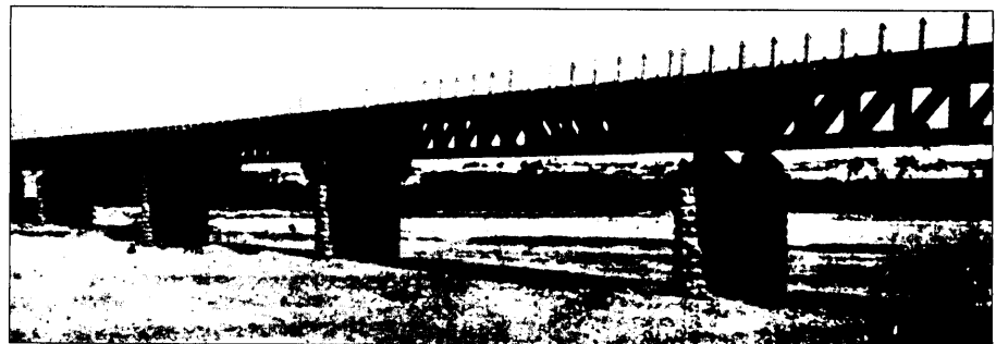
Figura 5: Puesto sobre el río Andarax en al provincia de Almería, compuesto por tramos de la colección oficial de Zafra (solución en celosía) con luces repetidas de 32 metros.
