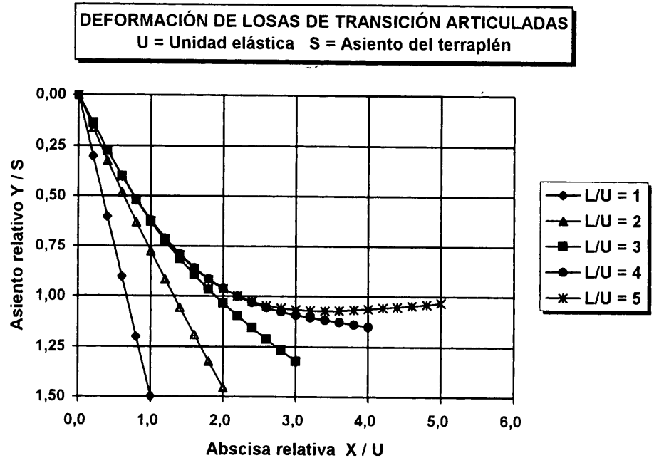
Figura 1. Deformación relativa de Losas de Transición Articuladas con diversas longitudes.
