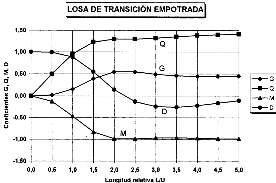
Figura 4. Coeficientes para determinar esfuerzos y corrimientos en Losas de Transición Empotradas.
