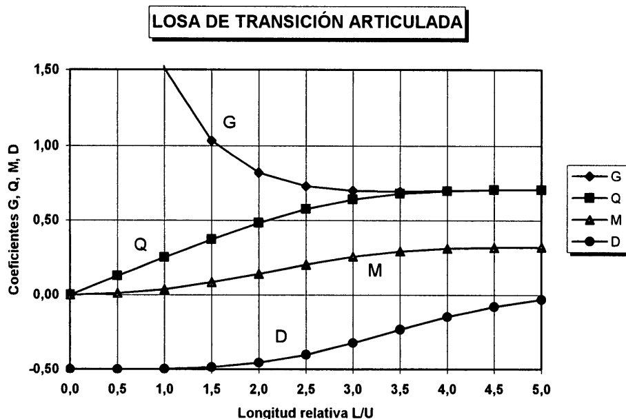
Figura 3. Coeficientes para determinar esfuerzos y corrimientos en Losas de Transición Articuladas.
