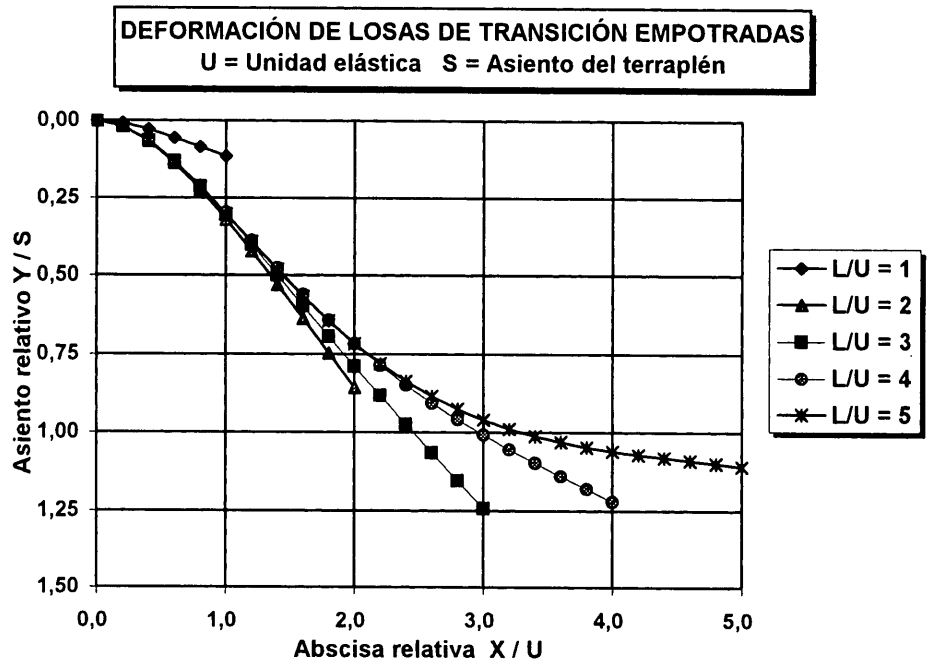
Figura 2. Deformación relativa de Losas de Transición Empotradas con diversas longitudes.
