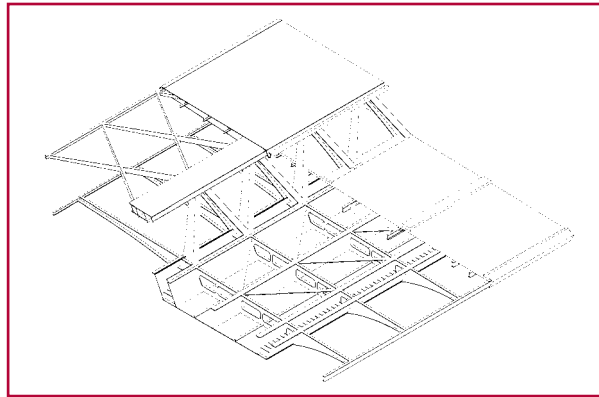
Fig. 2. Puente de Euskalduna. Bilbao. J. Manterola.
