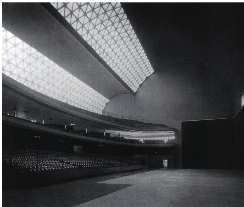
Fig. 5. Frontón Recoletos. E. Torroja.
