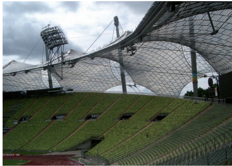
Fig. 4. Estadio Olímpico Munich. J. Schlaich.
