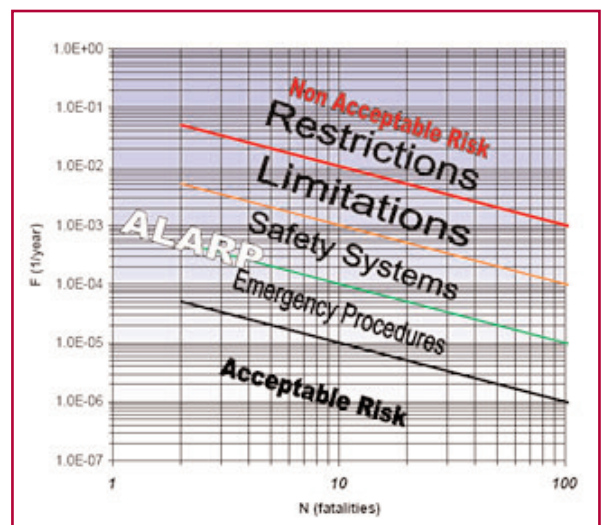
Fig. 12. Diagrama F-N donde se representa el riesgo social.
