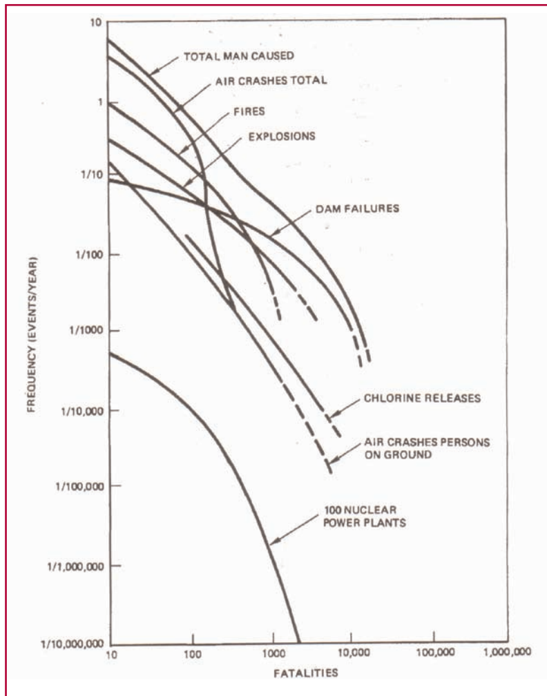
Fig. 1. Frecuencia de sucesos conducentes a N o más muertes.
