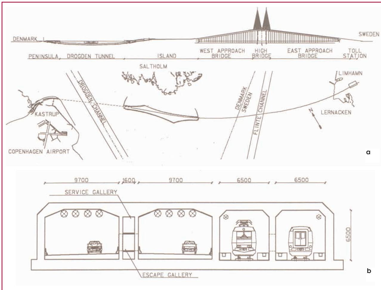
Fig. 2. a) sección longitudinal del túnel de 3,7 km bajo el canal Drogben. b) sección transversal de los tubos para el tráfico de carretera y ferroviario.
